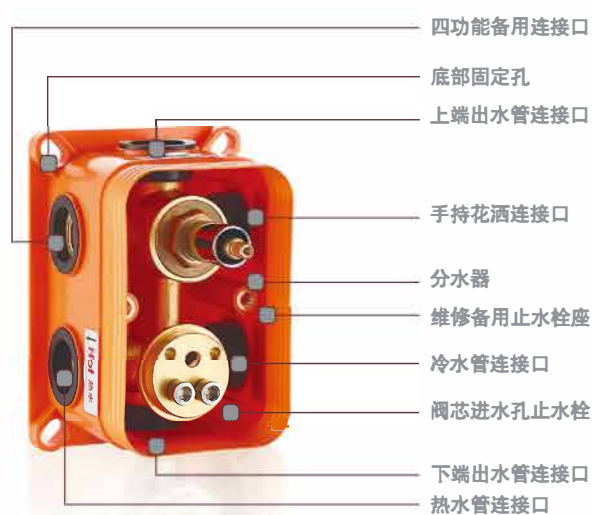
三功能连体式预埋盒
